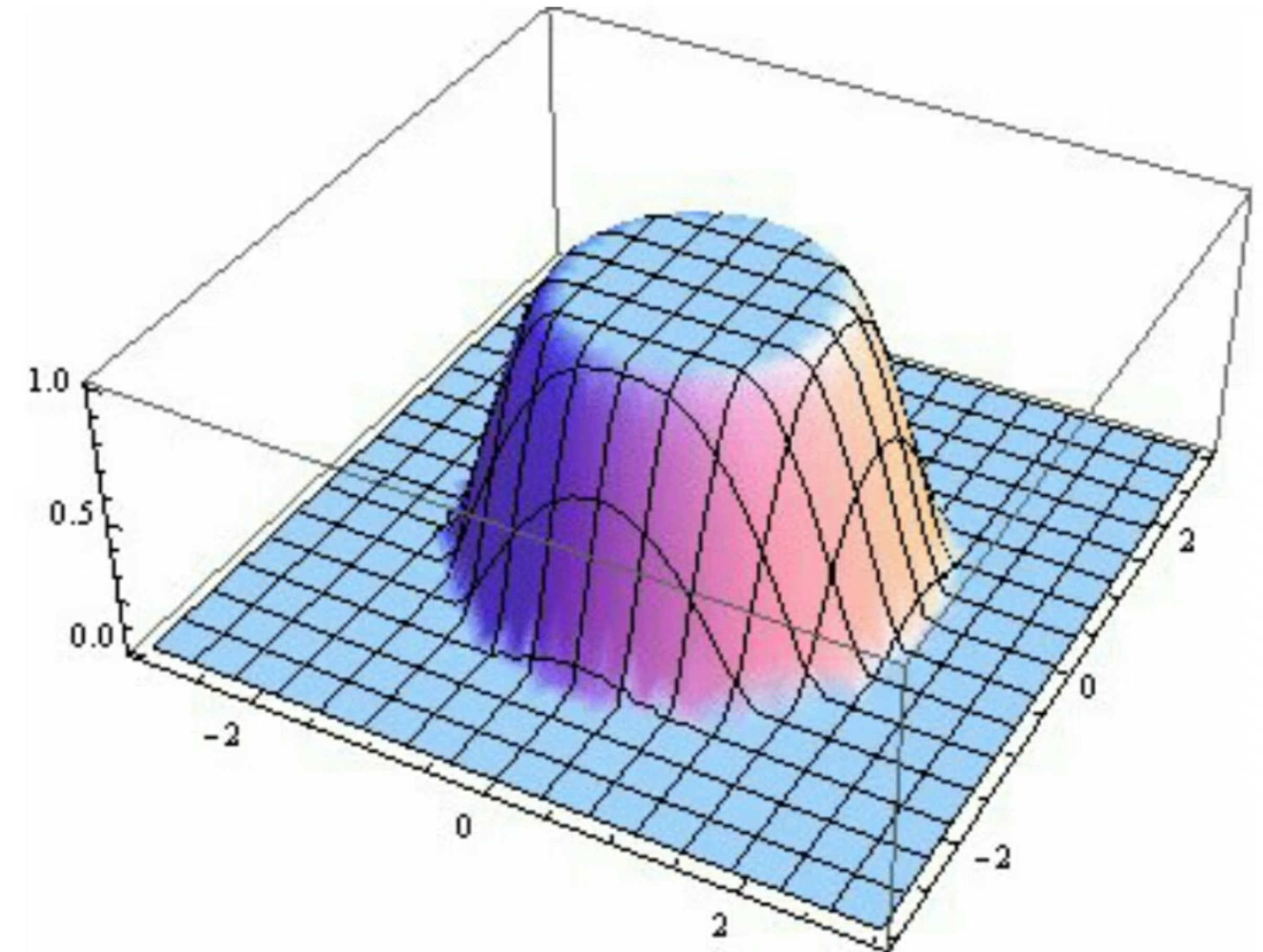
Rysunek 3. Wykres funkcji f(x_1, x_2) dla m = 2 . D_1 = \{(x_1, x_2) \in \mathbb{R}^2 : x_1^2 + x_2^2 \leq 1\} , D_2 = \{(x_1, x_2) \in \mathbb{R}^2 : x_1^2 + x_2^2 \leq 4\}
